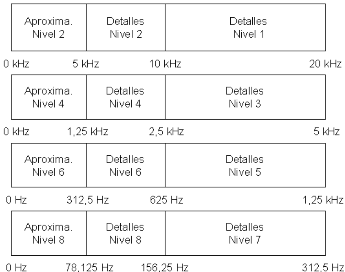
Figura 5.8. Distribución de Frecuencias por cada Escala o Nivel de la Descomposición. (Aproxima = Aproximaciones).
