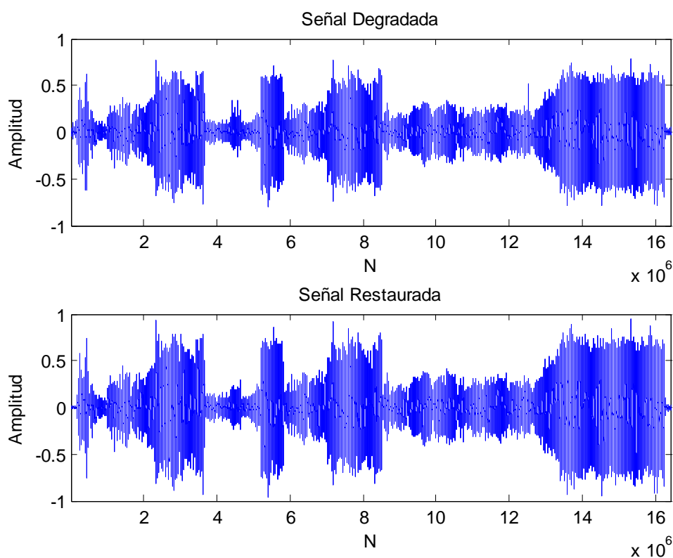
Figura 6.18. Comparación entre las Versiones Degradada y Restaurada de la Banda Sonora Waltz (Solamente el Canal Izquierdo).
