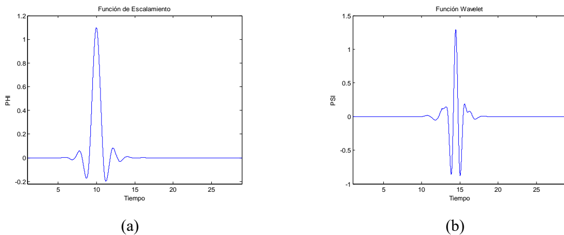
Figura 3.2. Coiflet de Quinto Orden. (a) Función de Escalamiento \phi(t) . (b) Función Wavelet \psi(t) .
